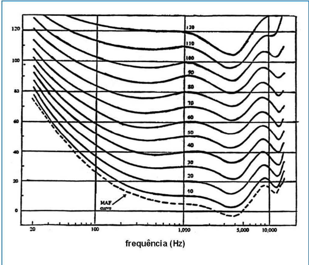
FIGURA 17 – CURVAS ISOAUDÍVEIS
