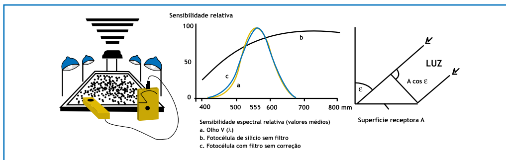
FIGURA 4 – LUXÍMETRO
